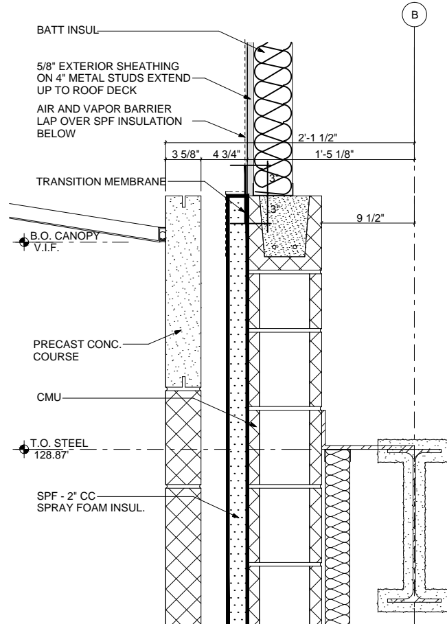
6 SECTION DETAIL A10.07 SCALE: 1"= 1'-0"
