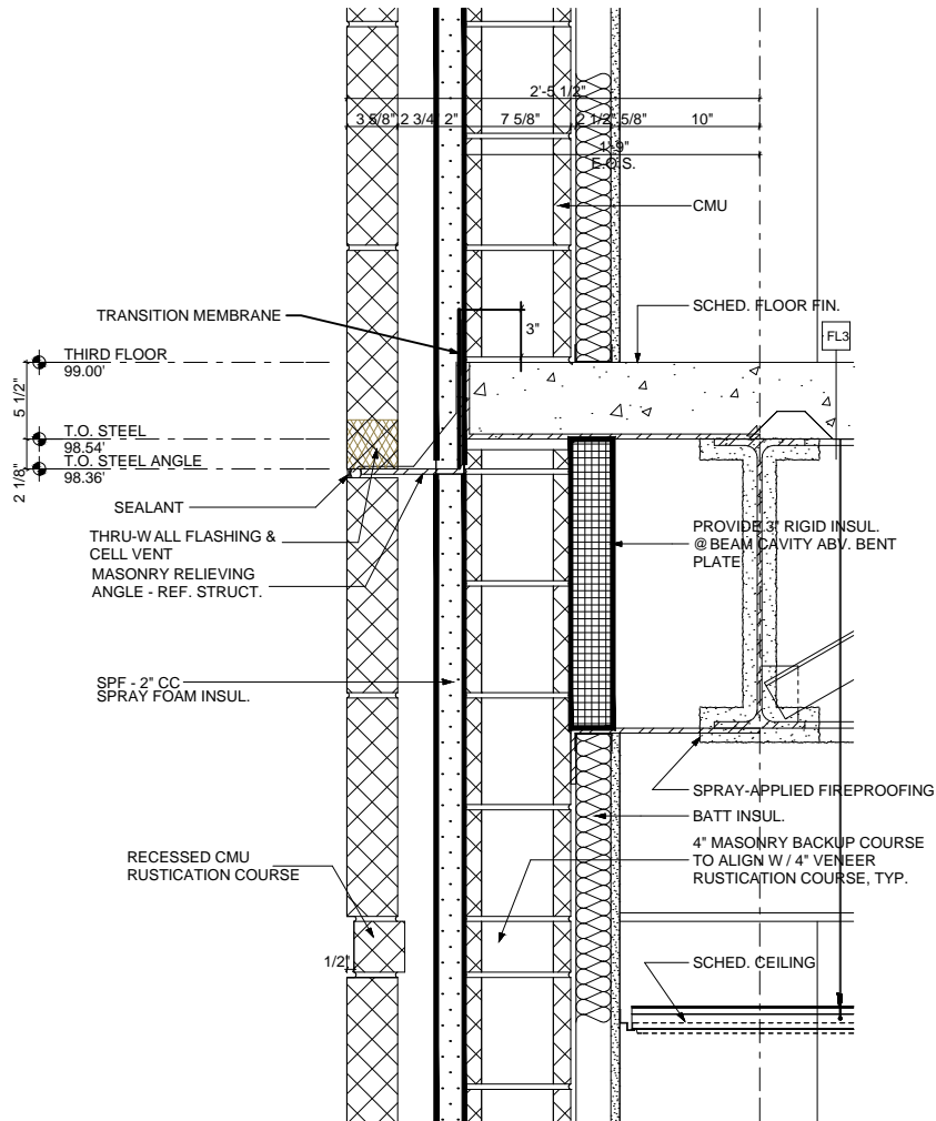
2 SECTION DETAIL A10.10 SCALE: 1" = 1'-0"
